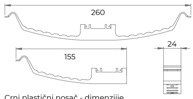
Crni plastični nosač - dimenzije nemontiranog nosača
