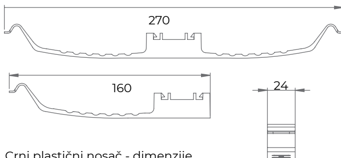
Crni plastični nosač - dimenzije montiranog nosača
